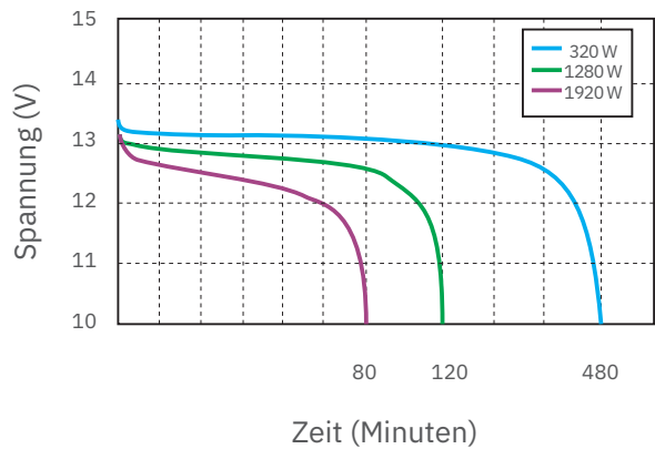
Konstante Leistungs- entladungseigenschaften (25 °C Umgebungstemp.)
