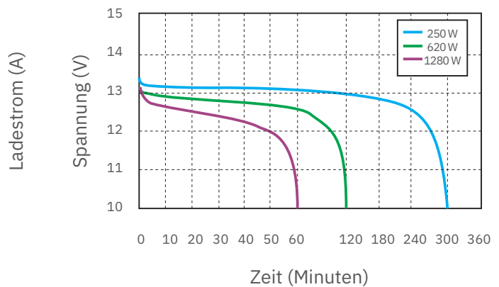
Konstante Leistungs- entladungseigenschaften (25 °C Umgebungstemp.)
